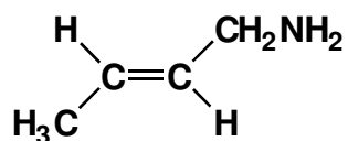
trans -2-Buten-1-amine
