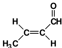
trans -2-Butenal
