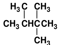
2,2,3-Trimethylbutane (bp 80.9°C)
