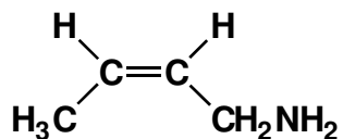
cis -2-Buten-1-amine
