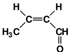
cis -2-Butenal
